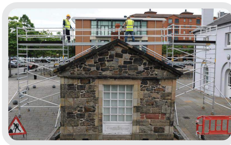
Spandek conecta 2 torres para el mantenimiento de la chimenea en Belfast.
